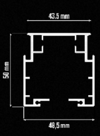
CODE: 13011 ** MOTORLU DİKEY PERDE ALÜMİNYUM RAYI
